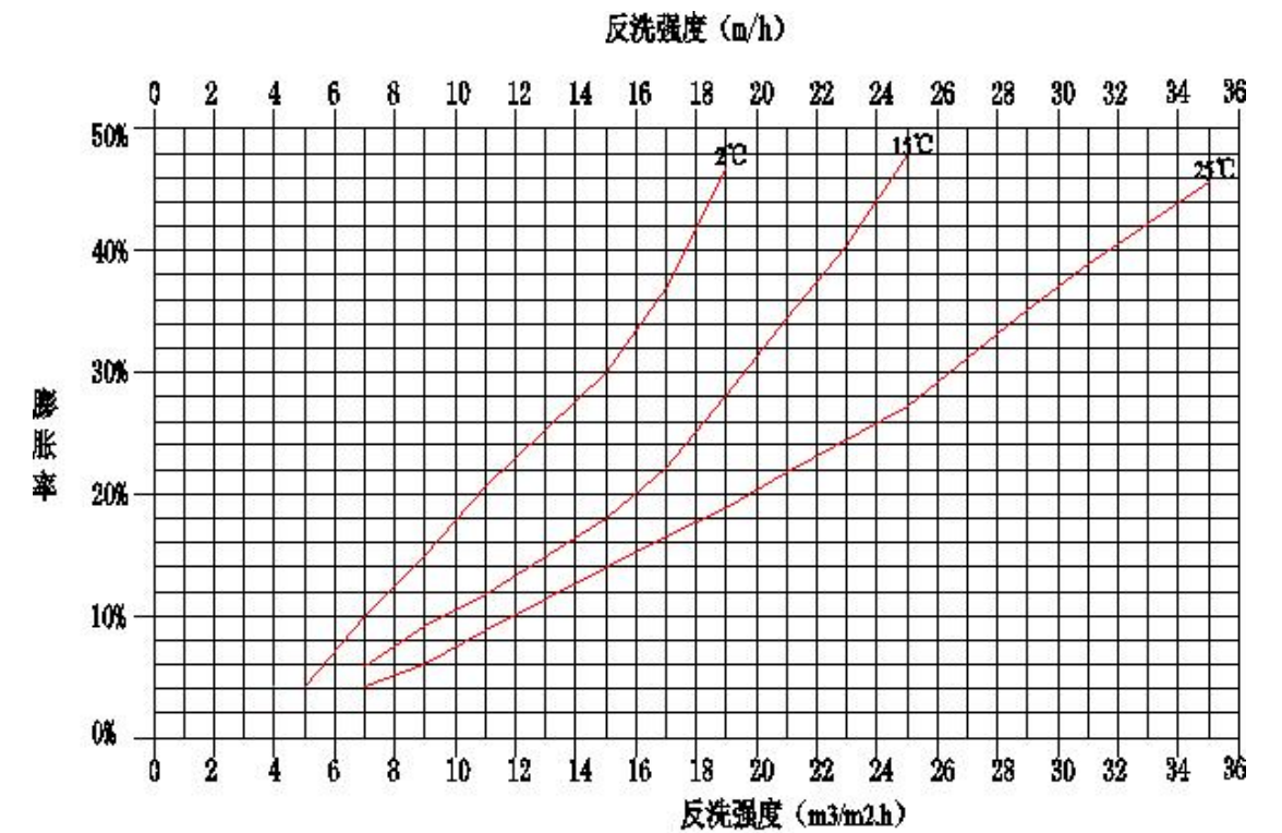
YTAC-165椰壳活性炭反洗强度与膨胀率关系图
